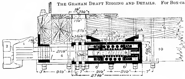
Fig. 1976. Longitudinal Section.
